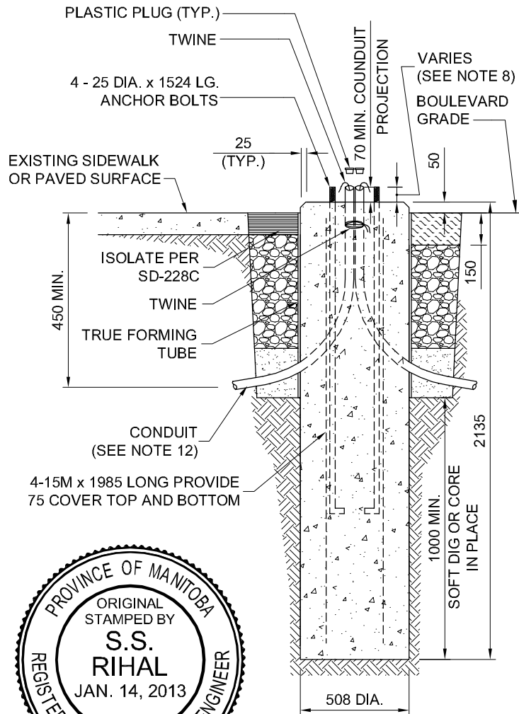
SECTION A-A
